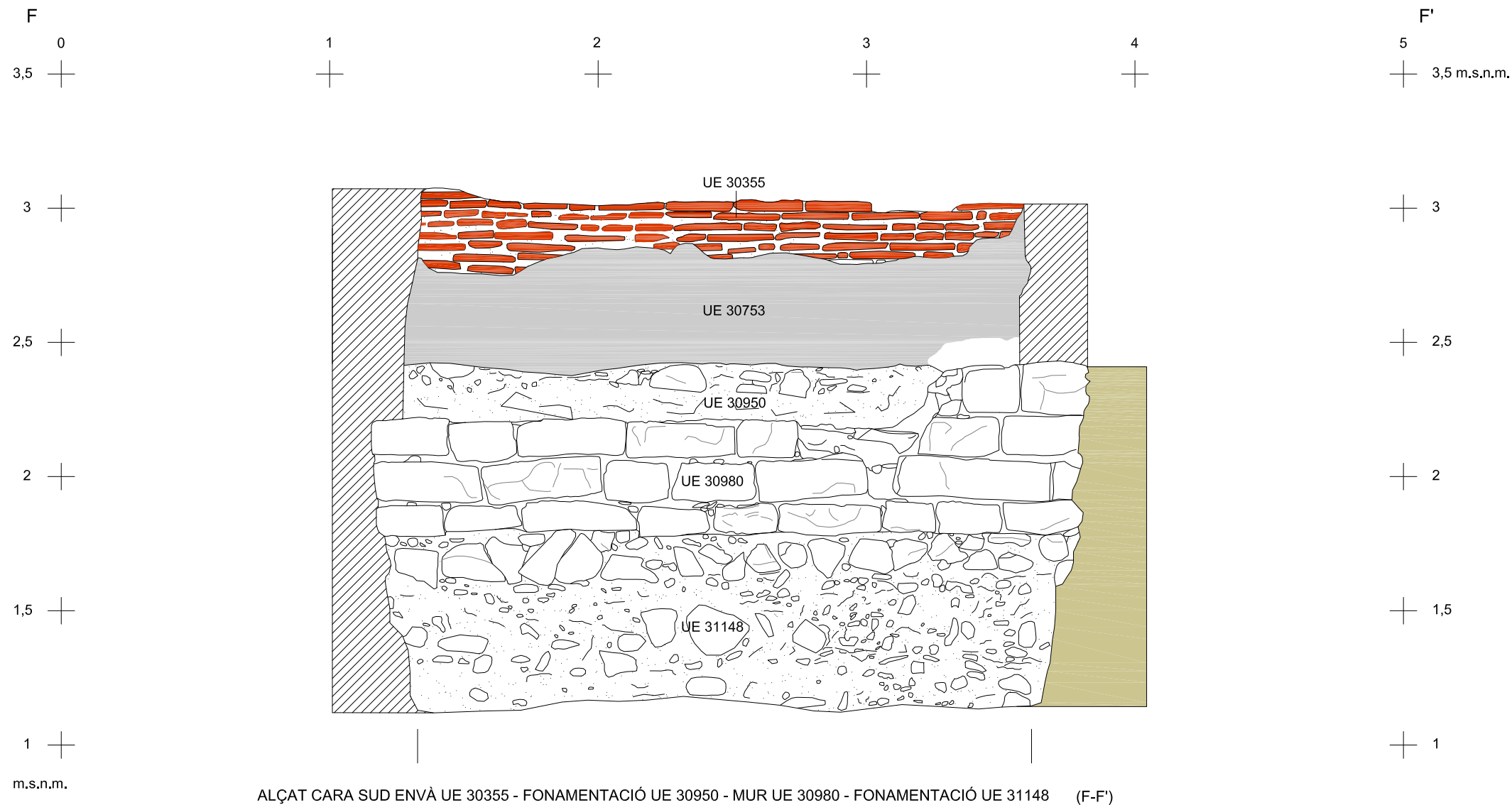
ALÇAT CARA SUD ENVÀ UE 30355 - FONAMENTACIÓ UE 30950 - MUR UE 30980 - FONAMENTACIÓ UE 31148 (F-F')
