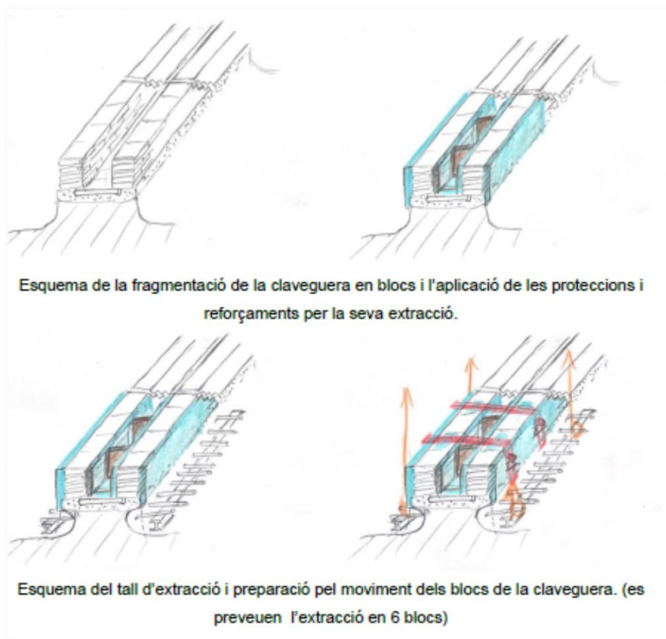
Proposta gràfica d'extracció seccionada de la claveguera (Àtics,SL-Gamarra i Garcia, Conservació-Restaureació)
