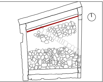
ALÇAT CARA NORD MUR UE 3980 - MENJADORA UE 30134 - MUR UE 31099 - FONAMENTACIÓ UE 31242 - REPARACIÓ UE 31133 (A-A')
