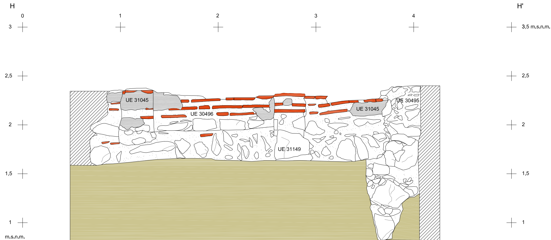
ALÇAT CARA OEST ENVÀ UE 30496 - FONAMENTACIÓ UE 31149 - FONAMENTACIÓ UE 30495 (H-H')
