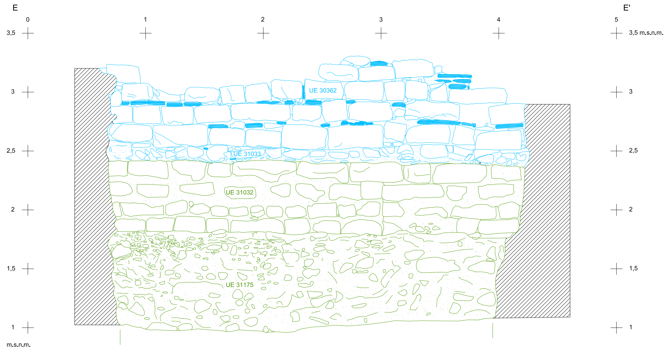
ALÇAT CARA NORD MUR UE 30362 - FONAMENTACIÓ UE 31033 - MUR UE 31032 - FONAMENTACIÓ UE 31175 (E-E')
