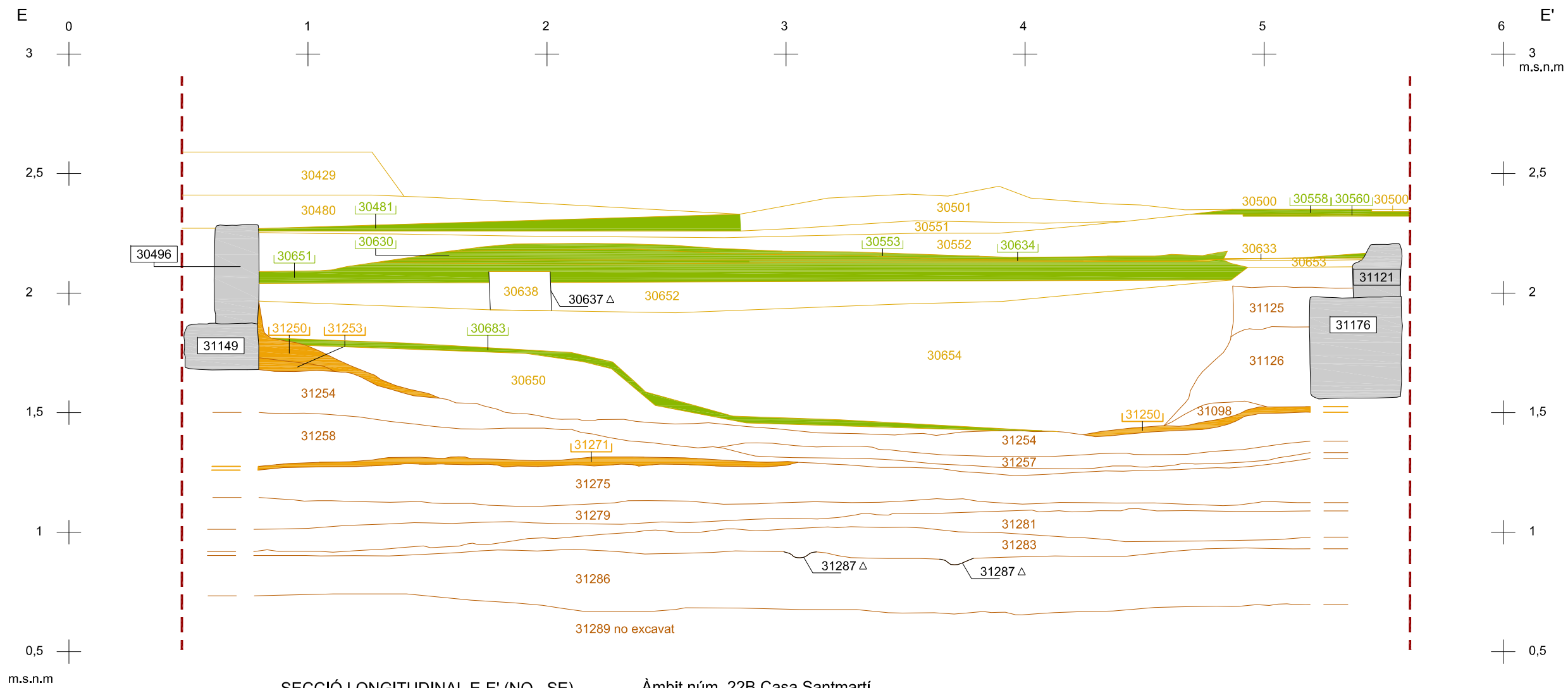
SECCIÓ LONGITUDINAL E-E' (NO - SE) Àmbit núm. 22B Casa Santmartí
