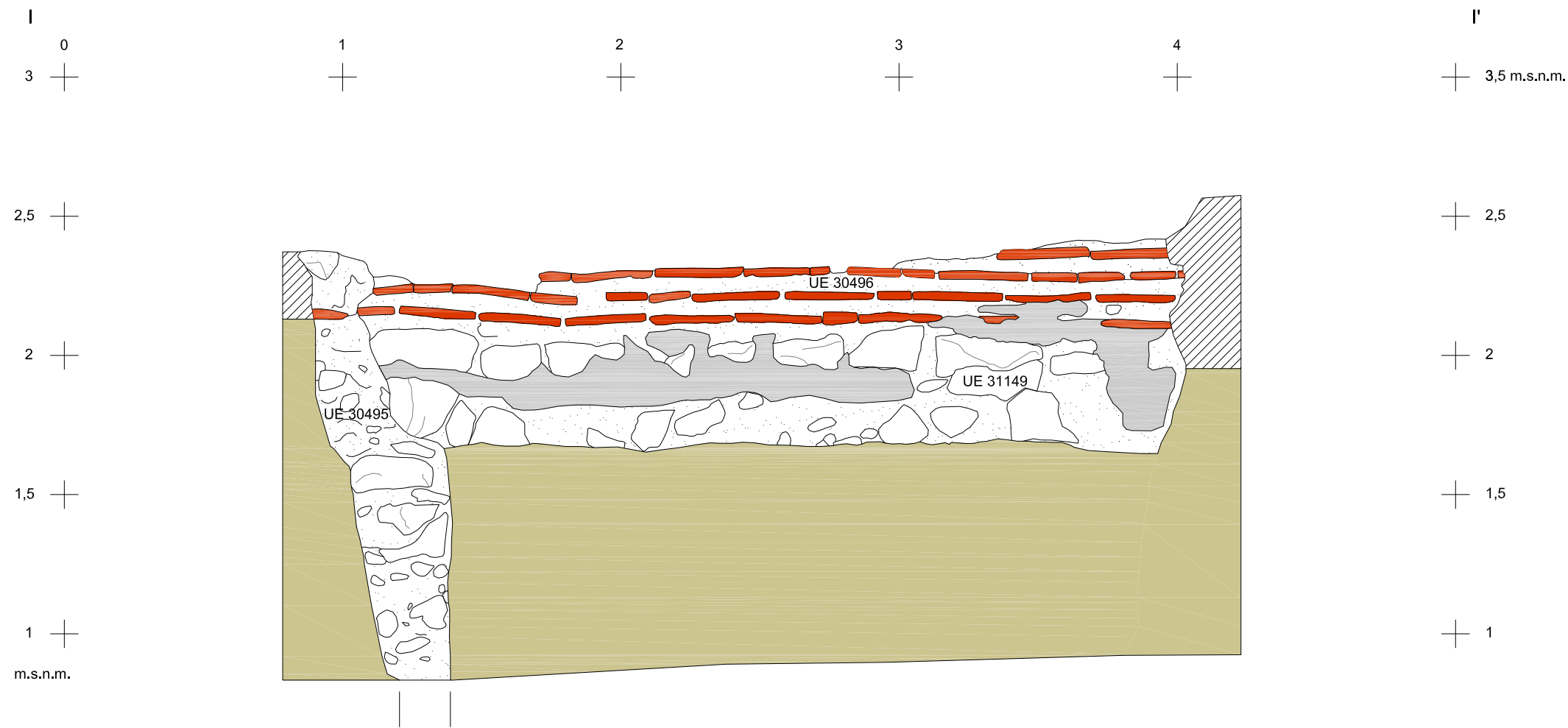
ALÇAT CARA EST ENVÀ UE 30496 - FONAMENTACIÓ UE 31149 - FONAMENTACIÓ UE 30495 (I-I')
